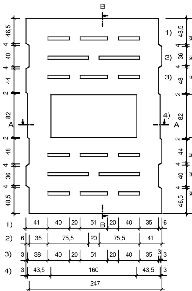
Untersicht
