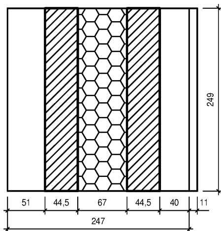
Schnitt A-A
