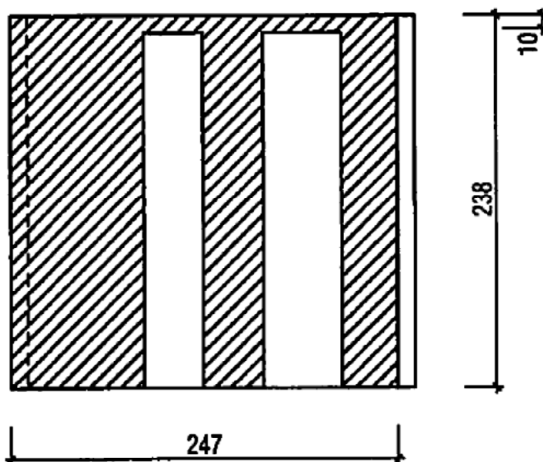
Schnitt 1 - 1
